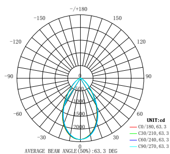
Beam angle: 60°
